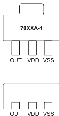
SOT-89
