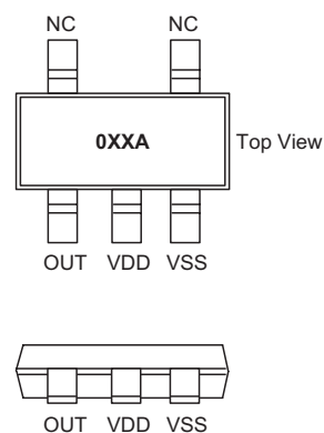
SOT-25
