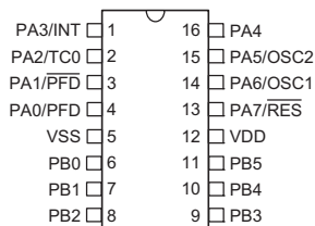
HT48R063 16 DIP-A/NSOP-A
