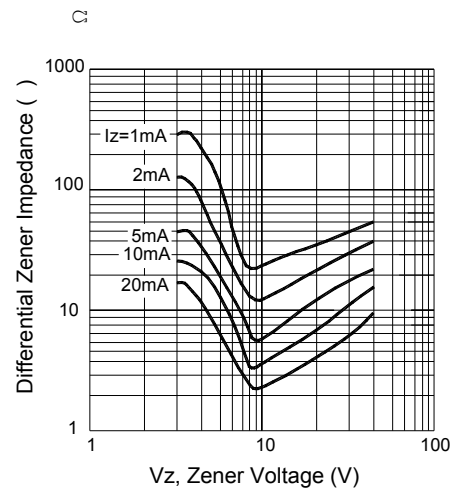
Fig. 4 Typical Zener Impedance vs. Zener Voltage
