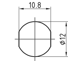
安装孔推荐尺寸
